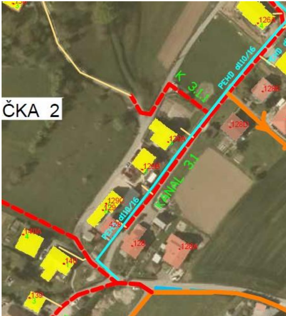
Območje Žitečka II.
