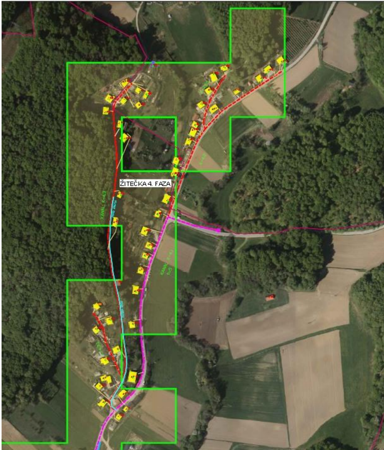
Območje gradnje kanalov K-4.1, K-4.2, K-4.2.1, K-4.3, K-4.3.1.
