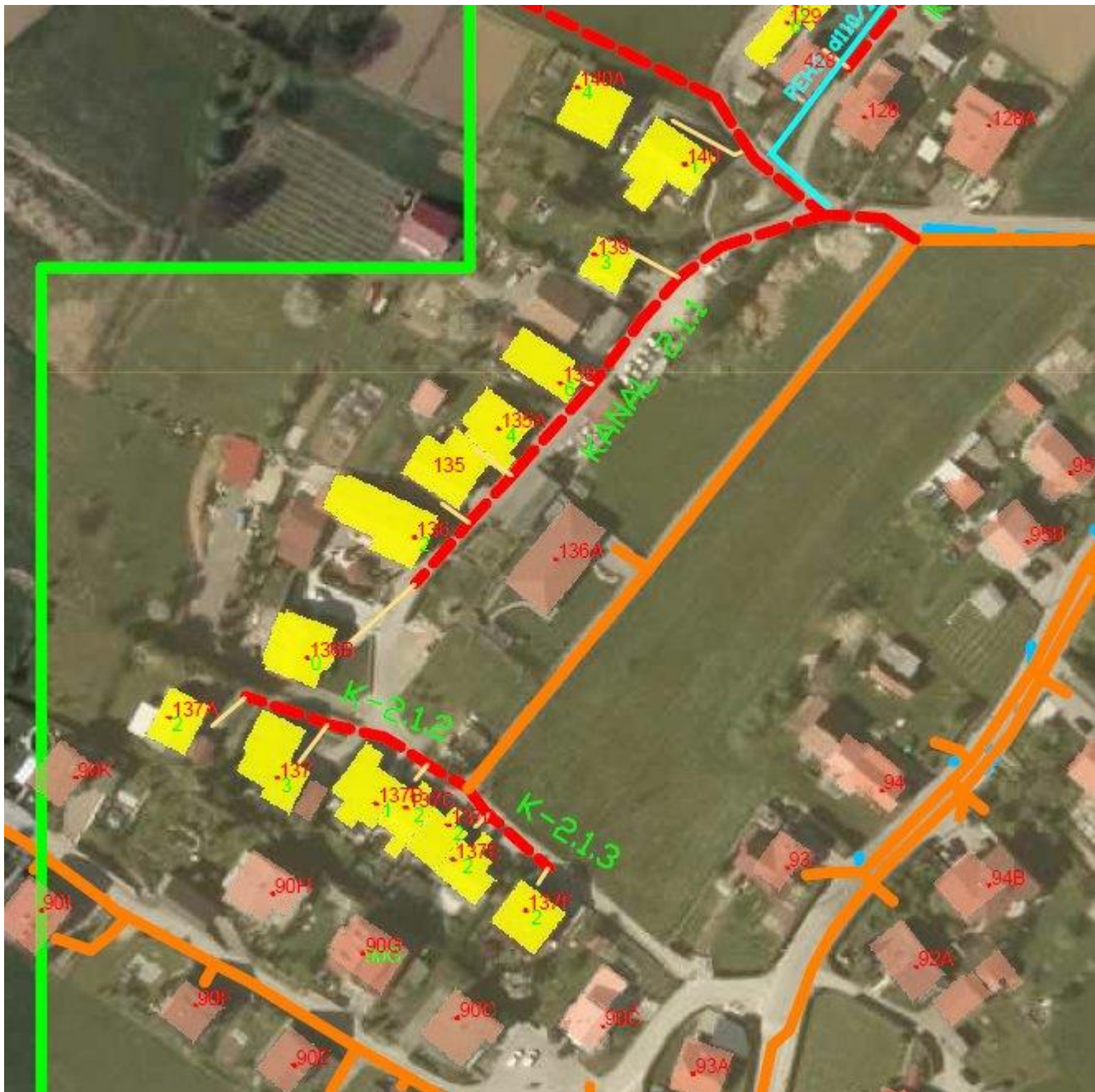
Območje gradnje kanalov K-2.1.1, K-2.1.2, K-2.1.3.
