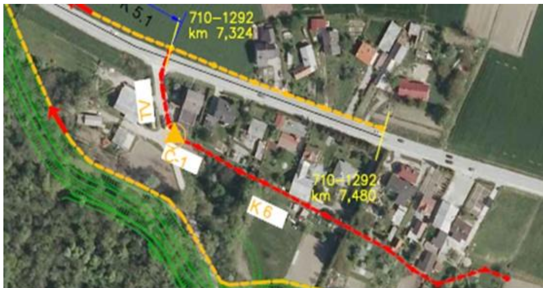
Lokacija gradnje kanala K-6.0.
